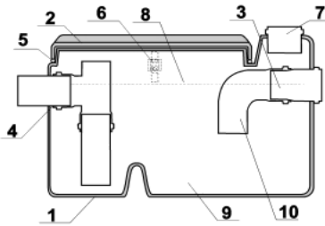
Принципова схема жироуловлювача серії СЖ "Оптиміа"
